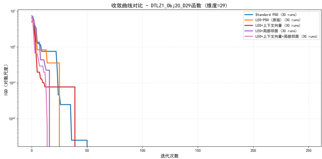
DTLZ1_20 目标收敛曲线
