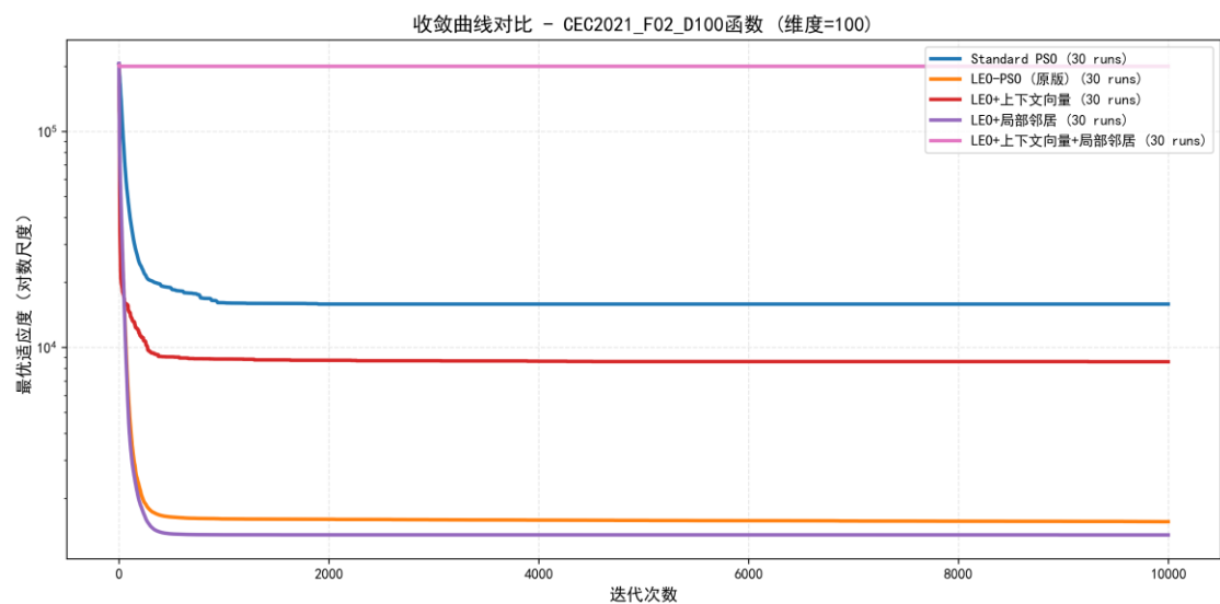
CEC2021_F02_D100 收敛曲线
