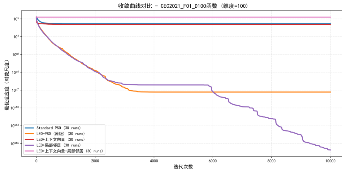
CEC2021_F01_D100 收敛曲线
