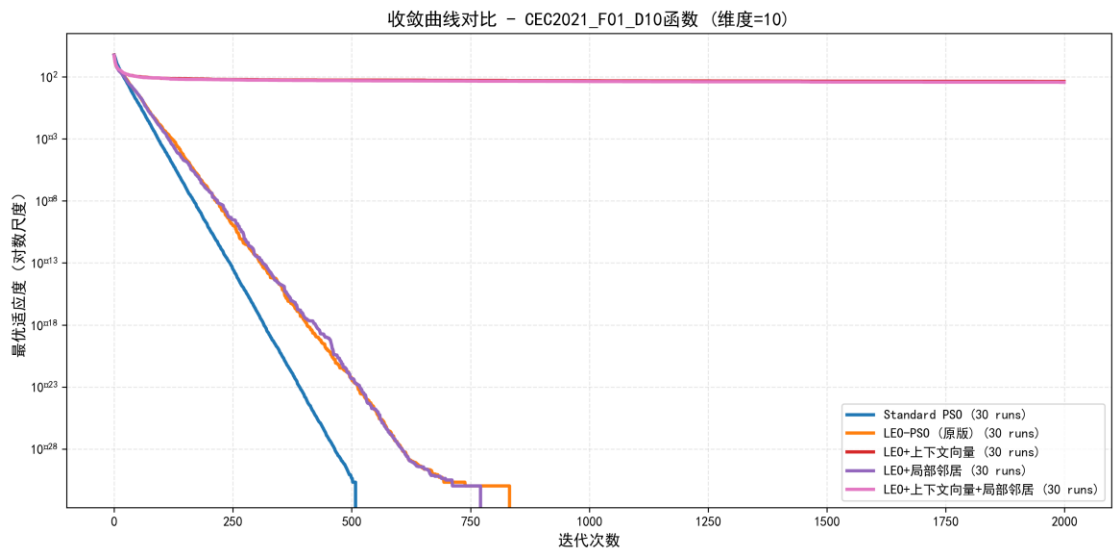
CEC2021_F01_D10 收敛曲线
