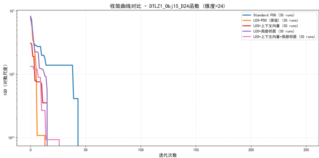
DTLZ1_15 目标收敛曲线
