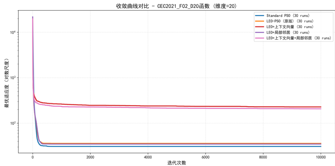
CEC2021_F02_D20 收敛曲线
