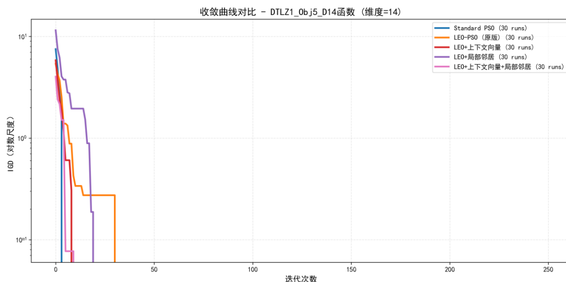
DTLZ1_5 目标收敛曲线
