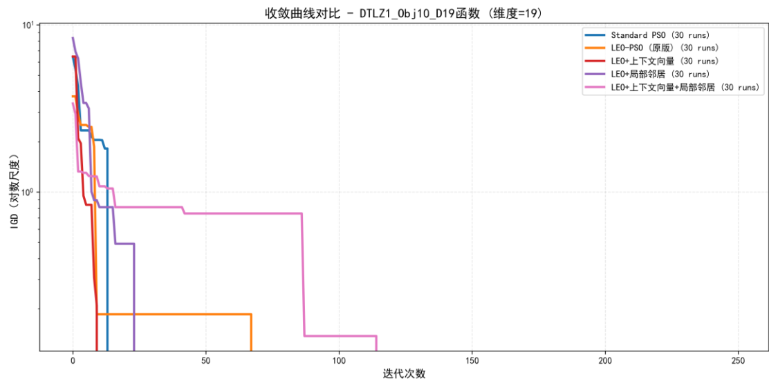
DTLZ1_10 目标收敛曲线
