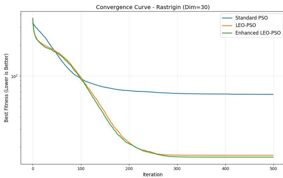
图 5.4.1 enhance_leo_pso (经验库大小 300)
